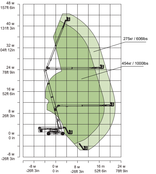
Диаграмма рабочей зоны ZA42J
